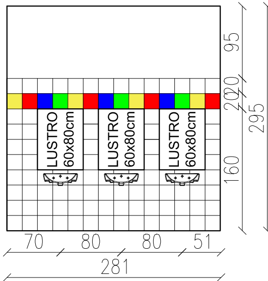
SCHEMAT RYSUNKOWY WYKOŃCZENIA ŚCIANY POMIESZCZENIA 0/01, PŁYTKAMI CERAMICZNYMI NIE GORSZYMI NIŻ PASTELE FIRMY TUBĄDZIN LUB RÓWNOWAŻNE
