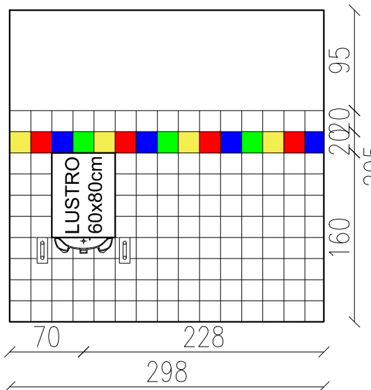
SCHEMAT RYSUNKOWY WYKOŃCZENIA ŚCIANY POMIESZCZENIA 0/04, PŁYTKAMI CERAMICZNYMI NIE GORSZYMI NIŻ PASTELE FIRMY TUBĄDZIN LUB RÓWNOWAŻNE
